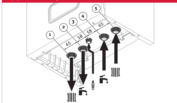
Připojení: kombinovaný kotel
